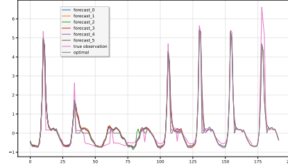
(d) 192-prediction on the Traffic dataset
