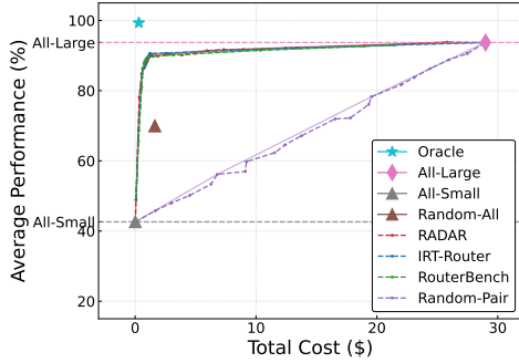
(e) LSAT
