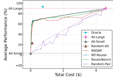
(f) AIME
