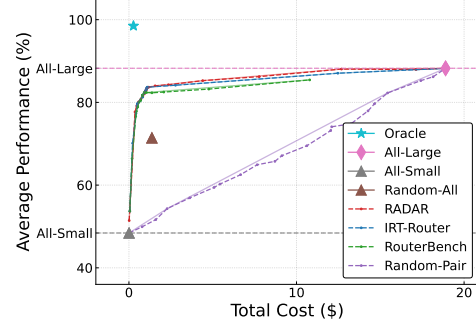
(b) MMLU
